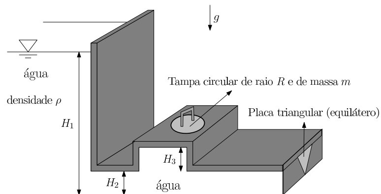
Figura 4.25: Sistema sob pressão.
