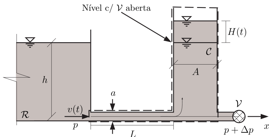
Figura 7.11: Oscilação num tanque devido ao fechamento abrupto de uma válvula.
