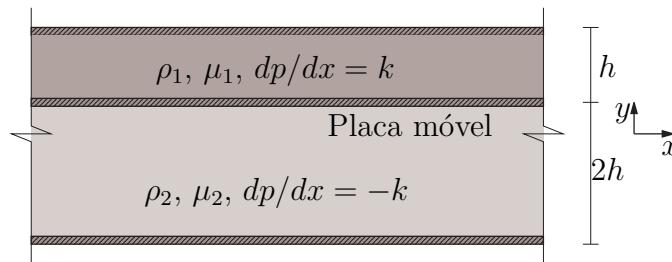
Figura 8.12: Dois fluidos e três placas.
