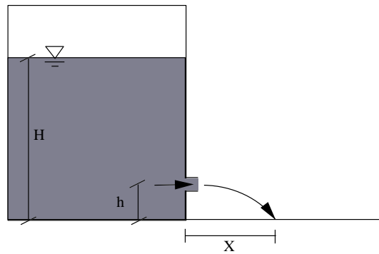
Figura 7.23: Tanque furado.
