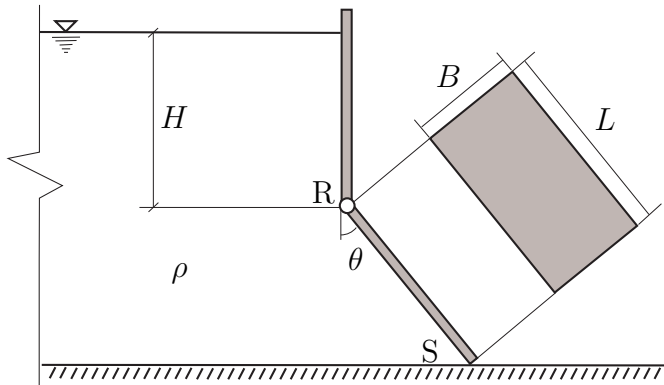
Figura 4.13: Comporta sujeita a pressão hidrostática.
