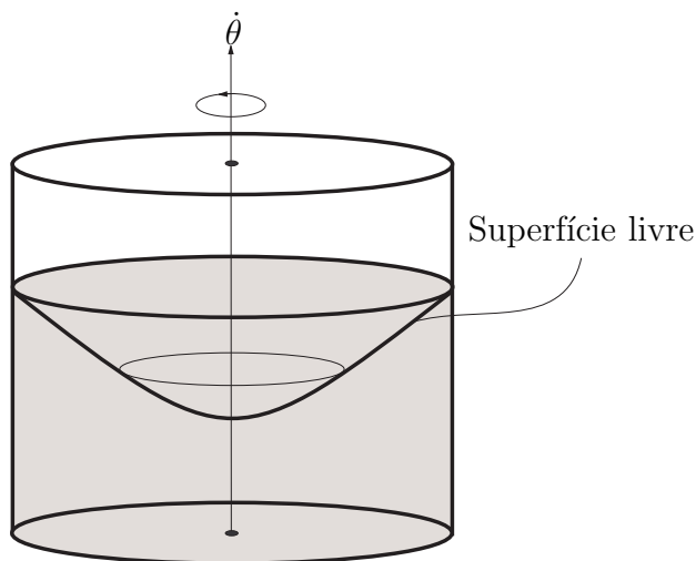
Figura 8.6: Fluido em rotação uniforme com superfície livre.
