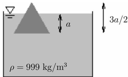
Figura 4.21: Bóia triangular.
