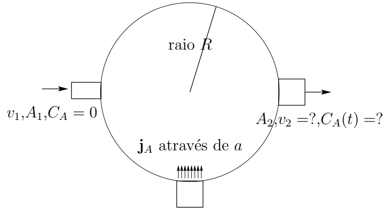
Figura 7.22: Esfera com soluto.
