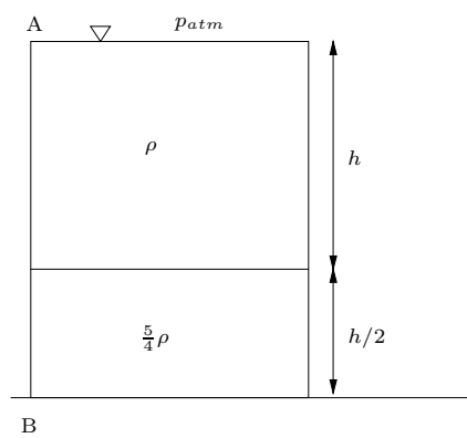
Figura 4.22: Pressão de 2 líquidos nas paredes de um tanque.
