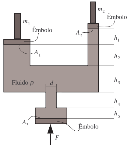
Figura 4.17: Sistema hidráulico em equilíbrio.
