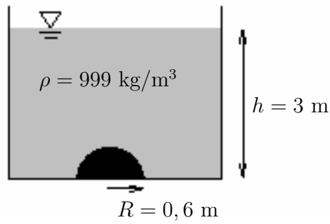
Figura 4.20: Força em calota hemisférica.
