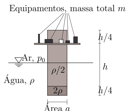
Figura 4.18: Bóia suportando equipamentos de medição.
