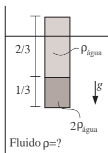
Figura 4.16: Problema da barra parcialmente imersa.
