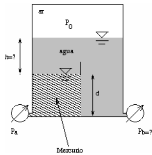
Figura 4.23: Pressão hidrostática.
