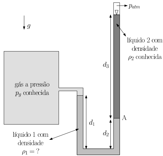
Figura 4.24: Tubo em U.
