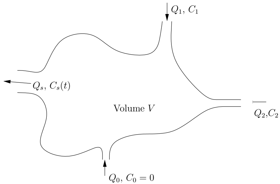
Figura 7.27: Lagoa com poluente.
